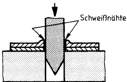
Verbinden der Werkstücke
