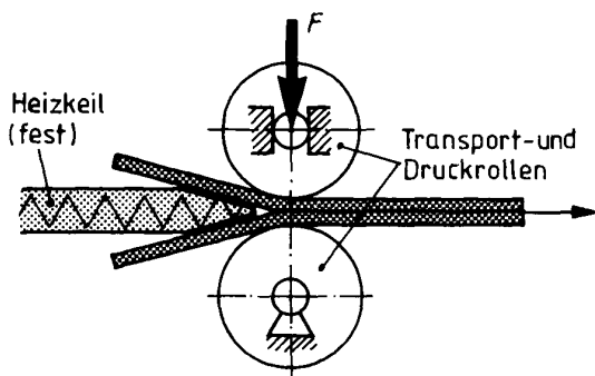
Heizkeilschweißen maschinell
