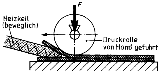
Heizkeilschweißen von Hand
